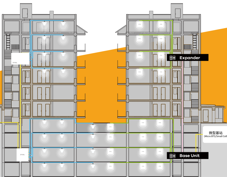
Repeater 強波器
